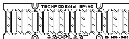
2 GRIGLIA IN GHISA D400 18 mm
