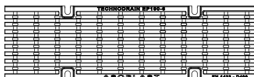
3 GRIGLIA IN GHISA D400 6 mm
