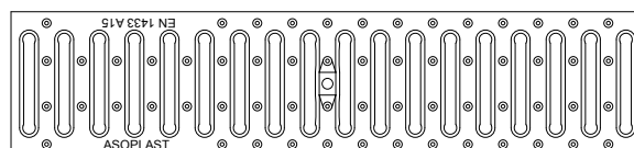
2 GRIGLIA A PIOLI ACCIAIO ZINCATO A15
