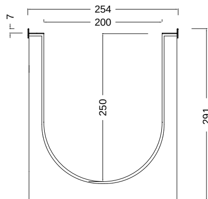
NEOMAX 200HV 200/250
